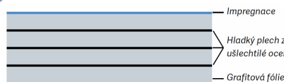
↑ Uspořádání vrstev
