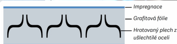
↑ Uspořádání vrstev
